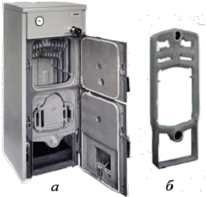
Вироби з легованих чавунів: а — котел; б — теплообмінник
